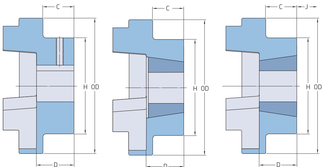
Typ B
