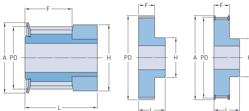
Typ OF
