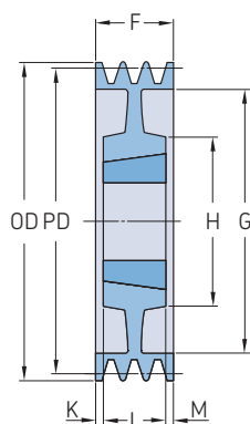
Typ 7
