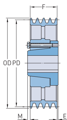
Typ C-3
