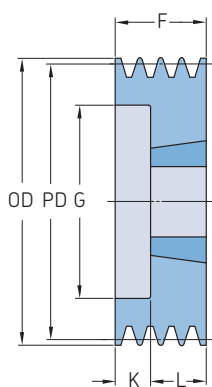
Typ 6
