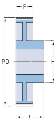
Typ 2
