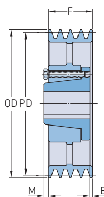
Typ B-3
