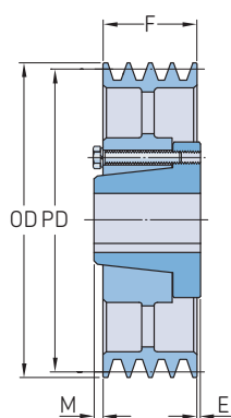
Typ C-3
