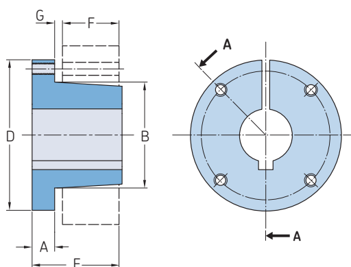
Velikost M-S
