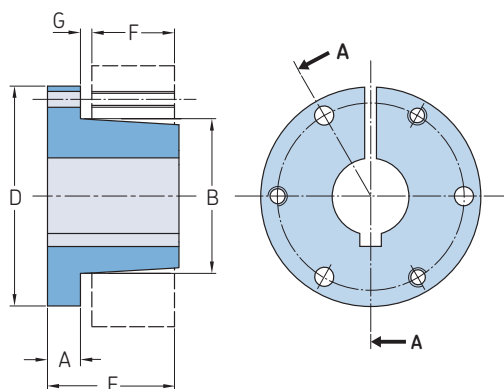
Velikost JA-J
