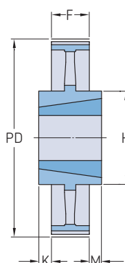
Typ 10
