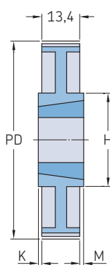
Typ 9
