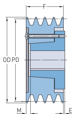
Typ D-1
