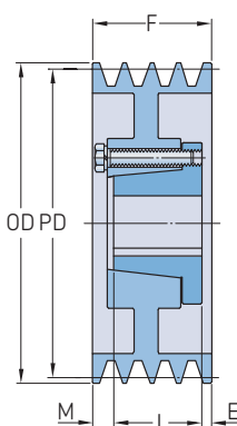
Typ A-2
