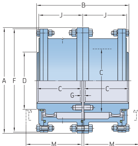
Velikost 80 až 120
