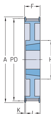
Typ 13F
