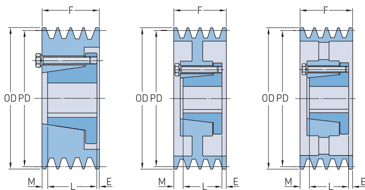
Typ A-1
