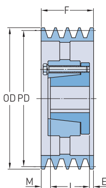
Typ A-3
