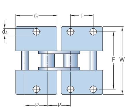
WK-1,WK-2
