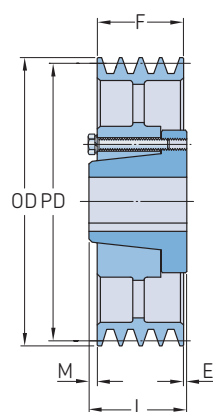
Typ C-3
