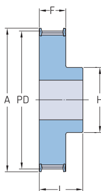
Typ 1F
