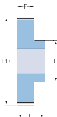
Typ 1
