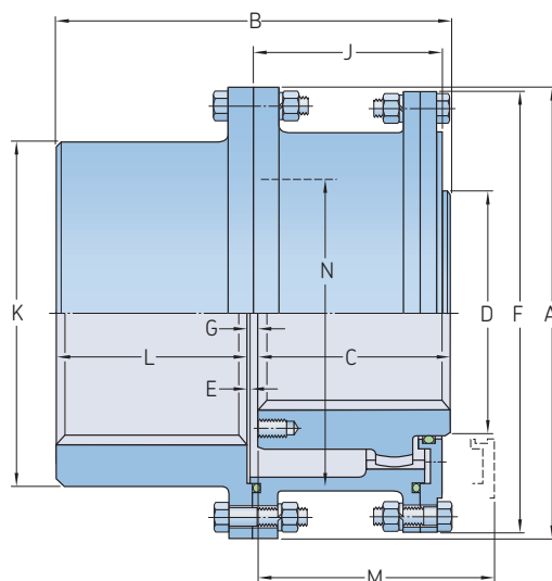
Velikost 80 až 120
