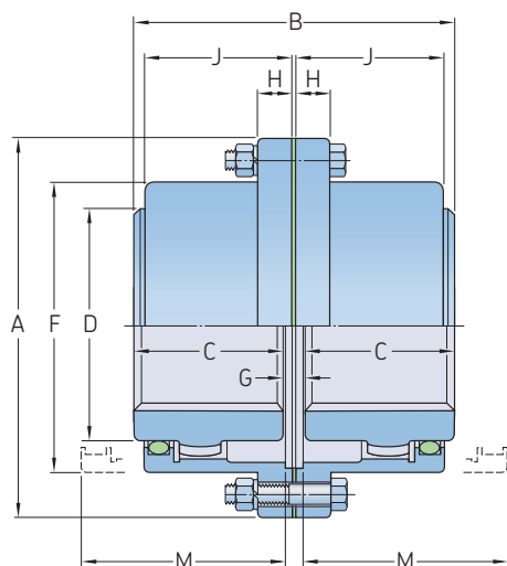
Velikost 10 až 70
