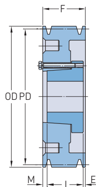
Typ A
