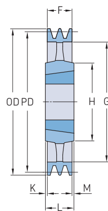
Typ 4
