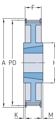
Typ 9F
