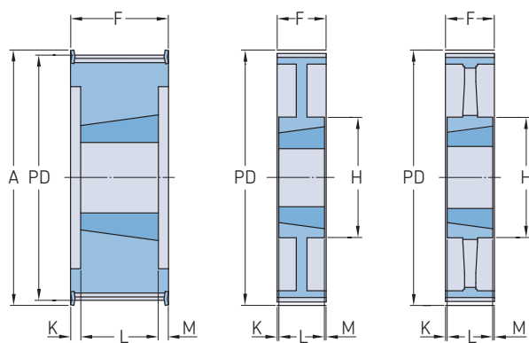
Typ 6F
