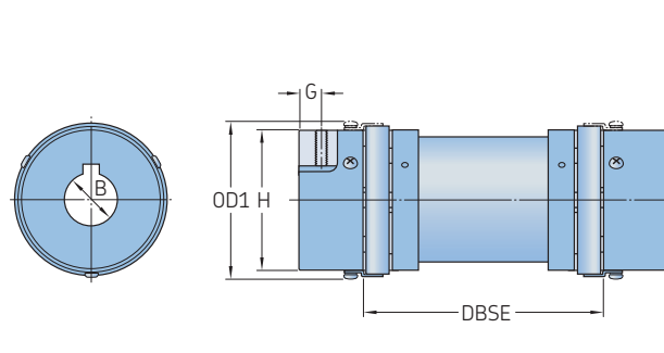
Rozpěrný díl
