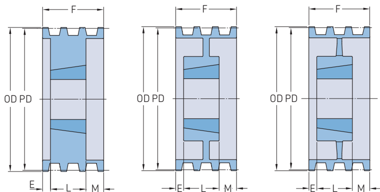
Typ A-1
