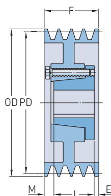
Typ A-2
