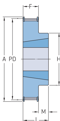
Typ 3F
