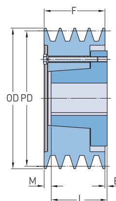
Typ D-1
